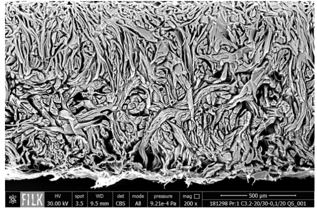
Abb. 1b: REM-Aufnahme, Querschnitt Kollagenvlies aus equiner Dermis
