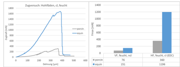
Abb. 2: Zugprüfung an Fadenmaterial. Fäden aus equinem Hautmaterial (blau) erreichen maximale Zugkräfte bis ca. 1200 mN (cl, vernetzt), porcine Fäden erreichen nur ca. 360 mN.
