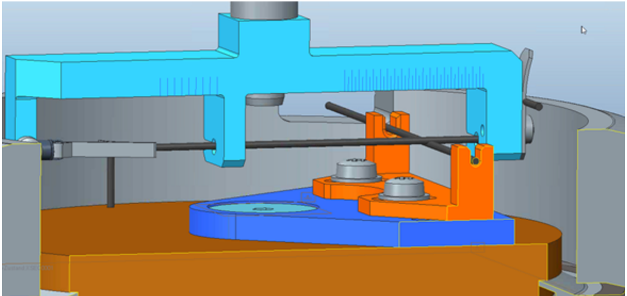
Abb. 1: Garnreibungsmessmodul
