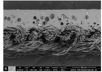
Abb.: REM-Querschnittsaufnahme eines mit rPVB-Compounds beschichteten PES-Gewirkes
