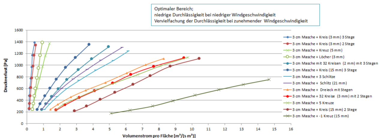
Abb. 2: Volumenstrom durch Verbunde, 3x3 cm, Druckverlust 200 – 1400 Pa
