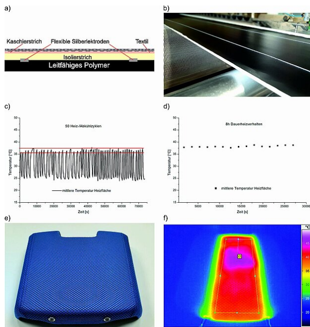
Abbildung: (a) Schichtaufbau der flexiblen, heizbaren Verbunde. (b) R2R-Herstellung von leitfähigen Folien mit aufgedruckten flexiblen Silberelektroden im technischen Maßstab. (c) Zyklisches Aufheiz- und Abkühlverhalten zeigt ein gleichbleibendes Temperaturniveau der heizbaren Verbunde in jedem Heizzyklus (markiert durch rote Linien). (d) Dauerheizverhalten über einen Zeitraum von 8 h mit einem konstanten Temperaturniveau über den gesamten Zeitraum. (e) Mit den im Projekt entwickelten heizbaren Verbunden wurde durch die Fa. Eissmann Automotive Deutschland GmbH eine Automobil-Armauflage als Demonstrator gefertigt. (f) IR-Abbildung der Armauflage bei 12 V Betriebsspannung
