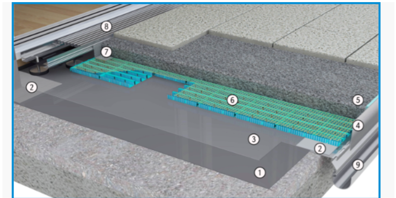
Abb.: Schematischer Aufbau eines Belagsystems (Ziffer 6 = Flächendrainage)
