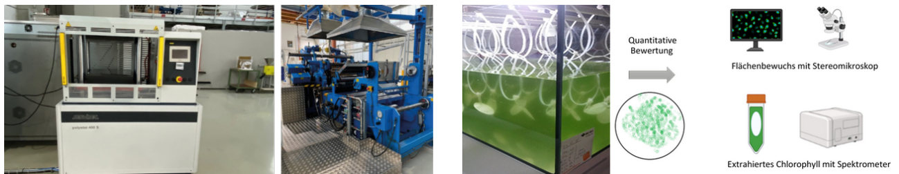
Abb. 1: Aufbringen der Mikrostrukturen mittels Heißprägen; links: diskontinuierlich (hydraulische Presse), rechts: kontinuierlich (Kalander)
