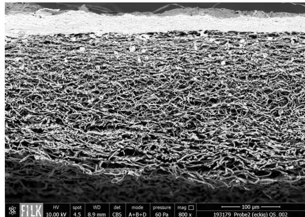
Abb. 2: REM-Aufnahme (800x) eines Pilzmycel-Composites
