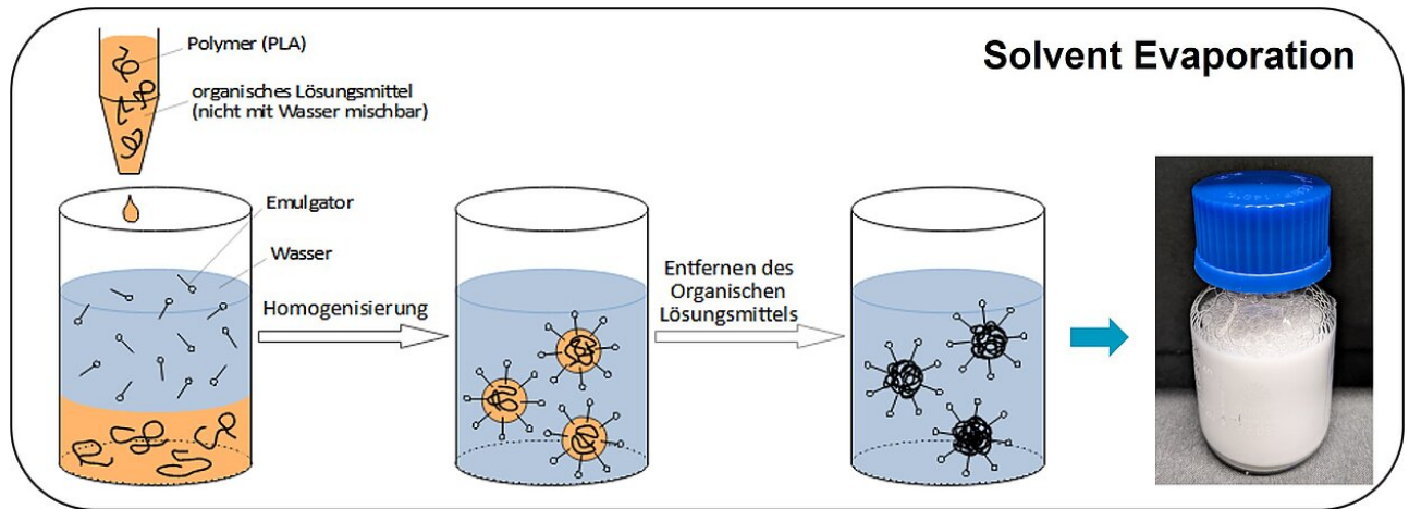
Abb.1.: Dispersionsherstellung über Methode Solvent Evaporation
