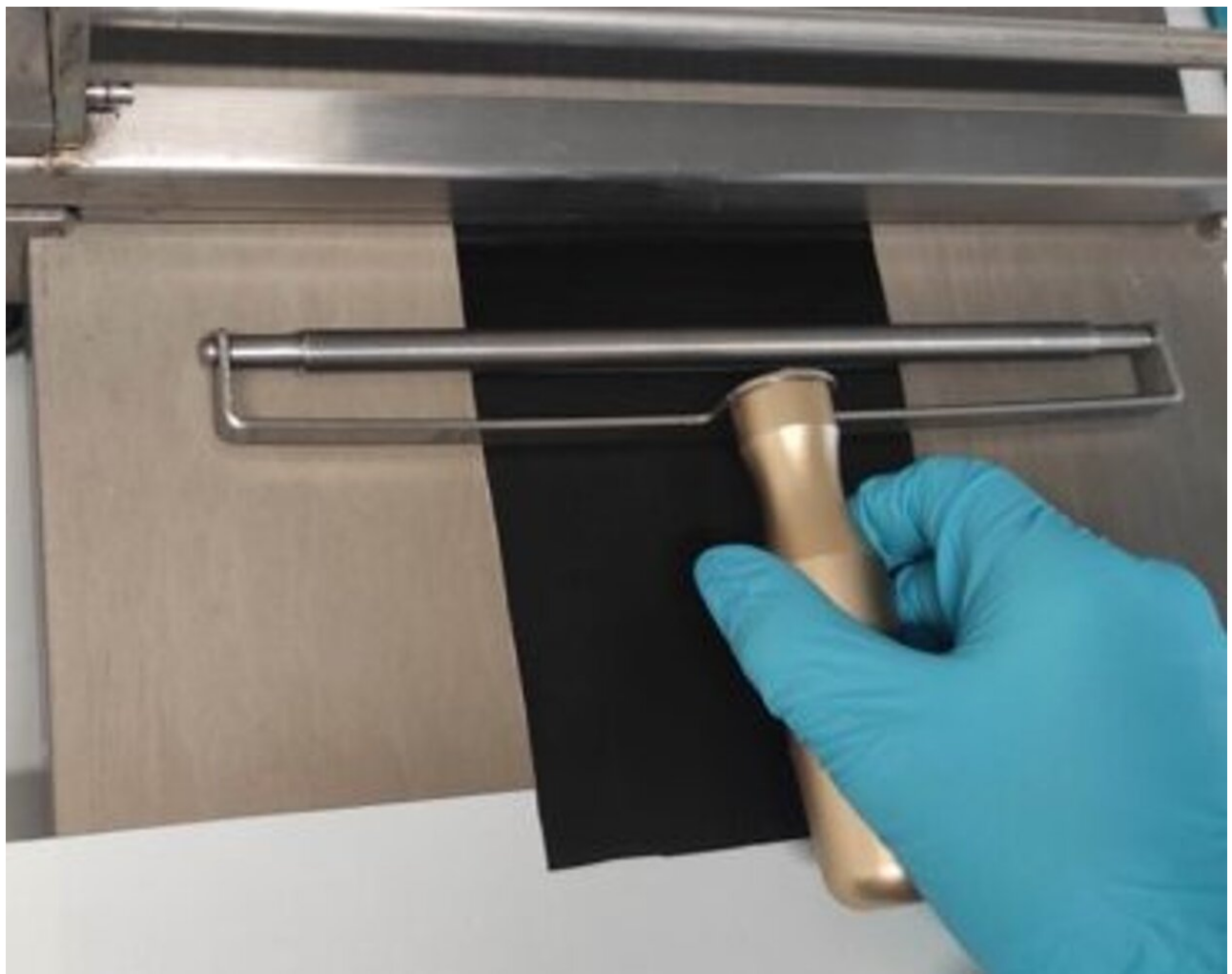
Abb.2.: Lackierung von PUR-Kunstleder mittels Spiralrakel
